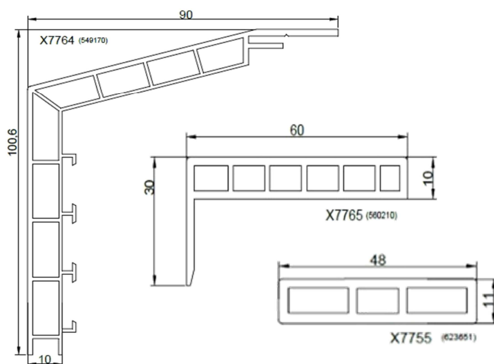
Battée arrondie, sur 2 vantaux Coloris standard
